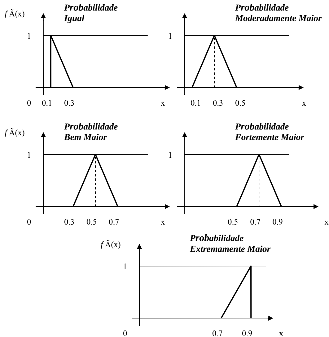
Figura 4. Representações Gráficas de Valores Fuzzy Triangulares da Variável Lingüística “Probabilidade de Perpetração da Ameaça”.
