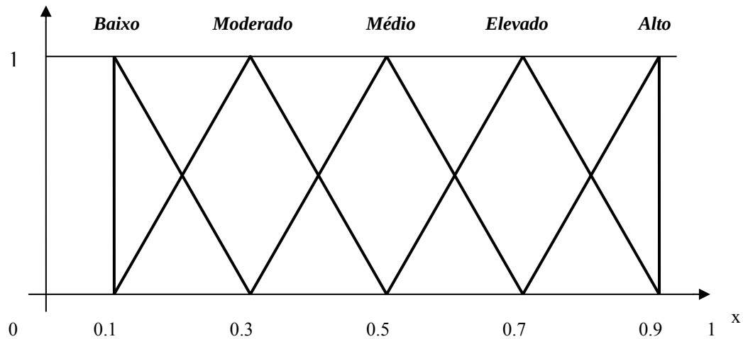
Figura 5. Números Fuzzy Triangulares Representativos da Variável Lingüística “Potencial de uma Ameaça Intencional a um Sistema de Transporte”
