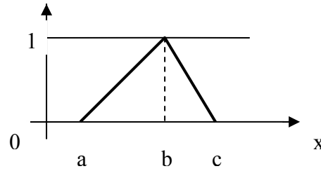
Figura 3 – Representação Gráfica de um Número Fuzzy Triangular
