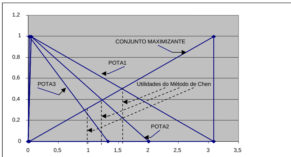
Figura 11: Método de Chen para Ordenar Números Fuzzy
