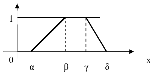
Figura 2 – Representação Gráfica de um Número Fuzzy Trapezoidal
