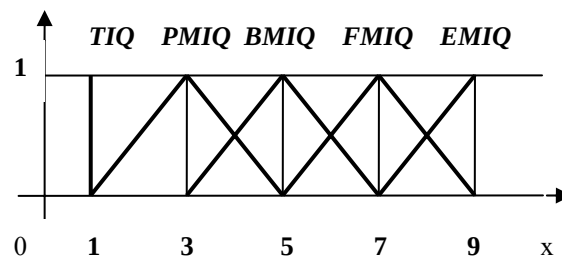
Figura 6 - Representação Gráfica dos Valores Lingüísticos da Variável Importância Relativa em Números Fuzzy Triangulares.
