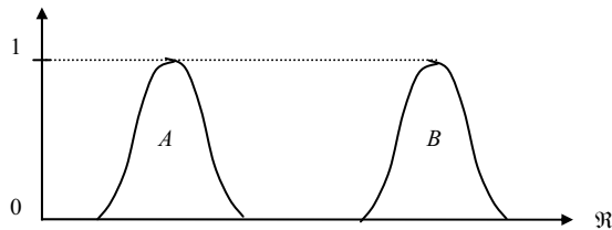
Fig. 6.10. Fuzzy interval
